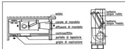
Esempio di ventilconvettore installato nel controsoffitto. Sez. trav. di un ventilconvettore a doppia batteria per impianto a quattro tubi.
