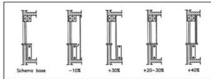
Effetto della posizione dei tendaggi sulla resa termica di un radiatore.
