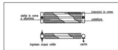
Schema di batteria alettata
